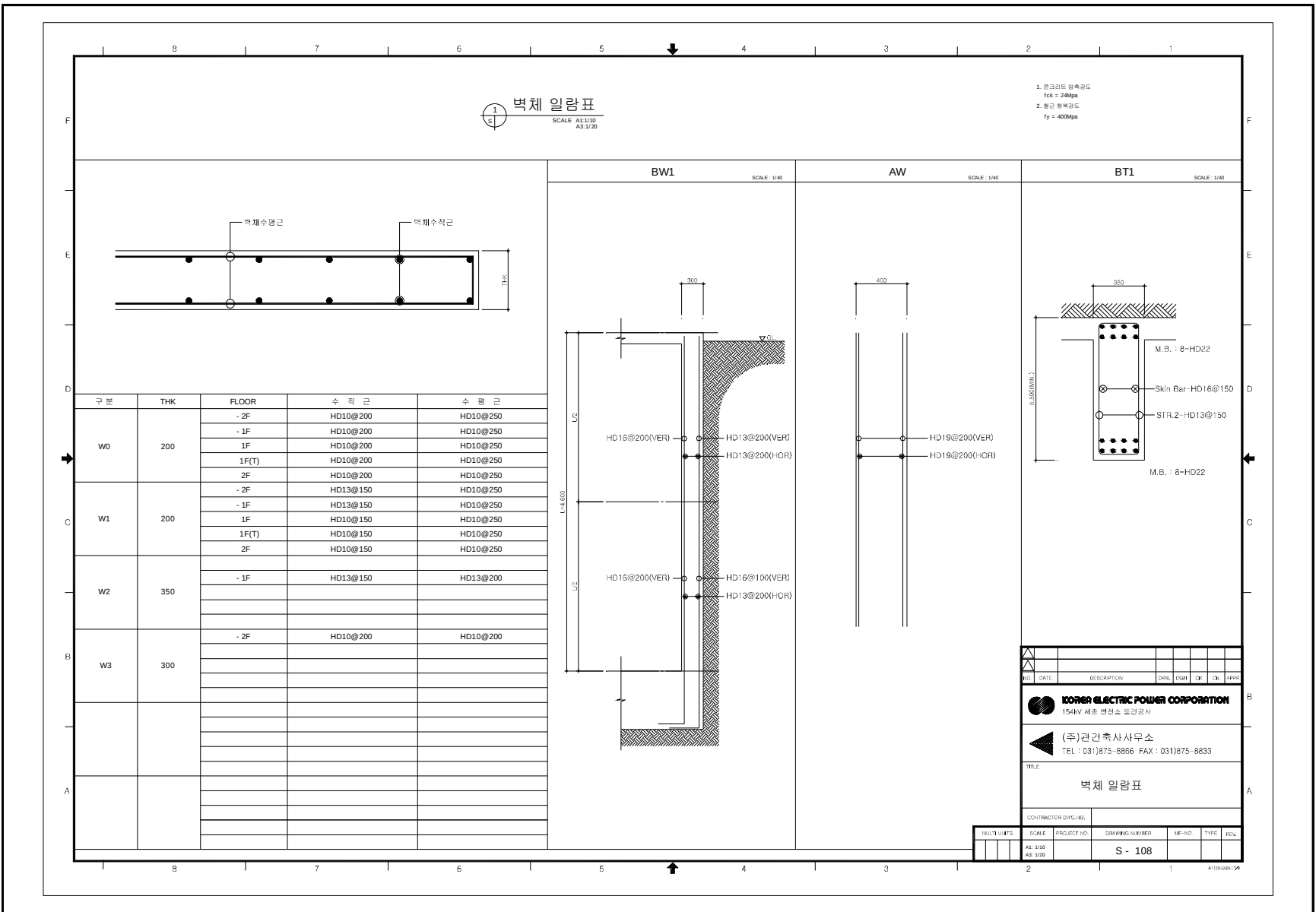
【그림 1.1.7】 RC옹벽 철근 배근도
