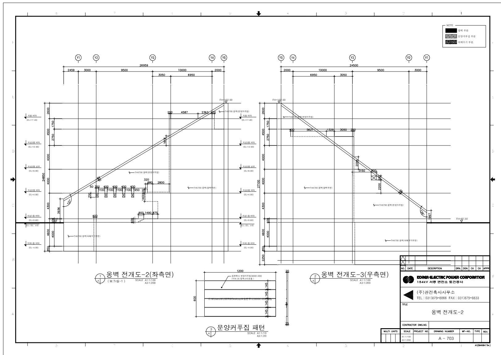
【그림 1.1.6】 RC옹벽 전개도(계속)
